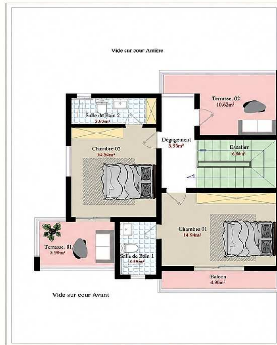
PLAN ETAGE
