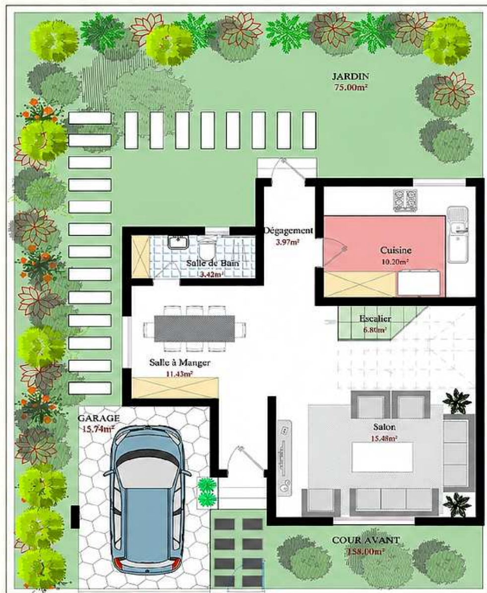
PLAN RDC
